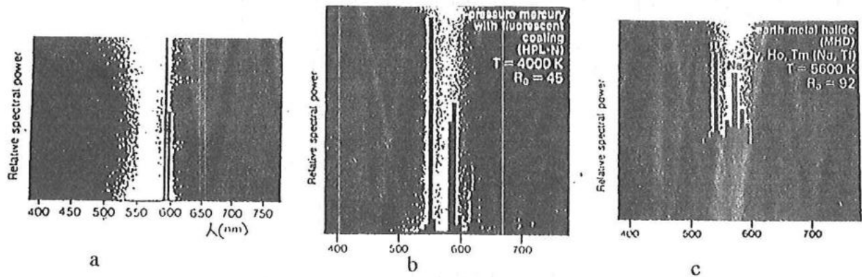
Figura 6 Structura emisie spectrale pentru surse cu: a – descărcări în sodiu la j.p.; b – idem mercur î.p. și balon fluorescent, c – M.H.
