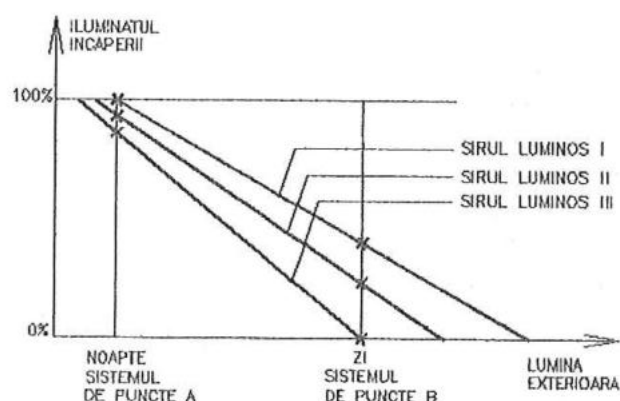
Figura 3 Caracteristicile de reglaj ale sistemului LUXMATE-DAYLIGHT
